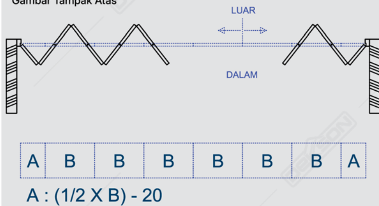
Gambar Tampak Atas
