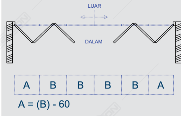
Gambar Tampak Atas
